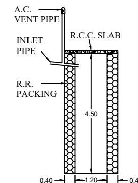
SOAK PIT
