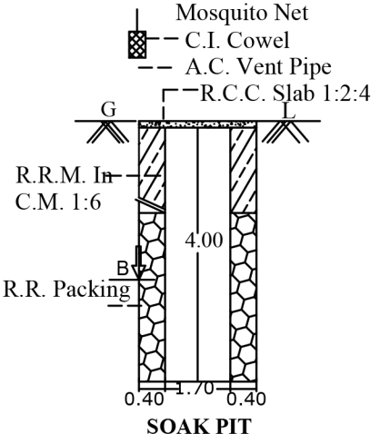
SOAK PIT
