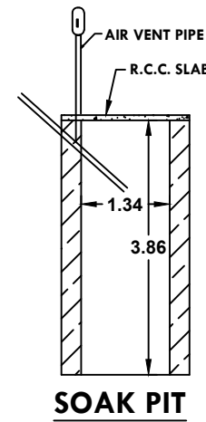
SOAK PIT
