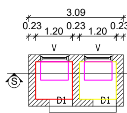
TOILET PLAN
