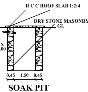
SOAK PIT
