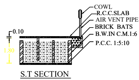
S.T SECTION
