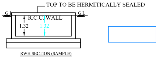
RWH_CAPACITY_L=4800LTRS
