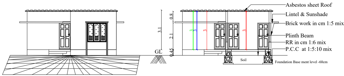
SECTION A-A
