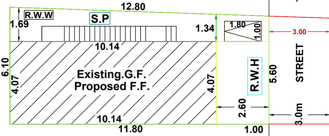
SITE PLAN SCALE 1:100
