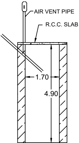
SOAK PIT
