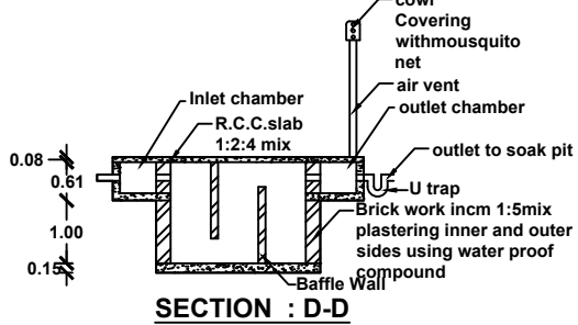
SECTION : D-D
