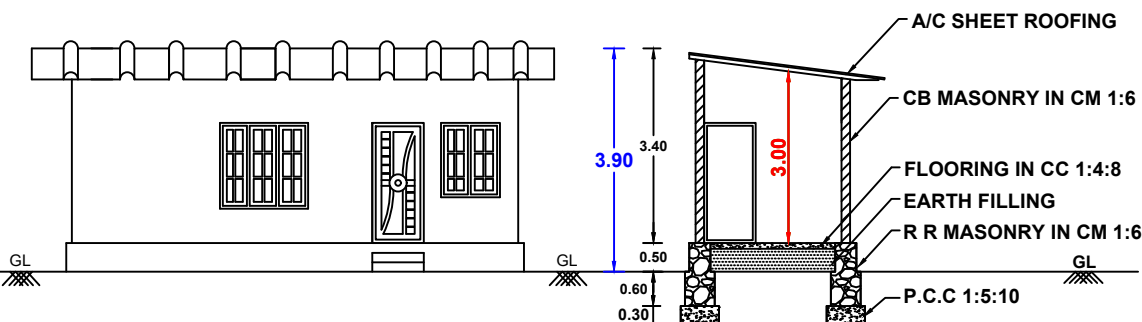
ELEVATION
