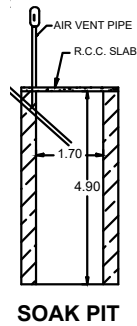
SOAK PIT
