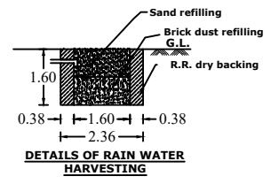
SOAK PIT
