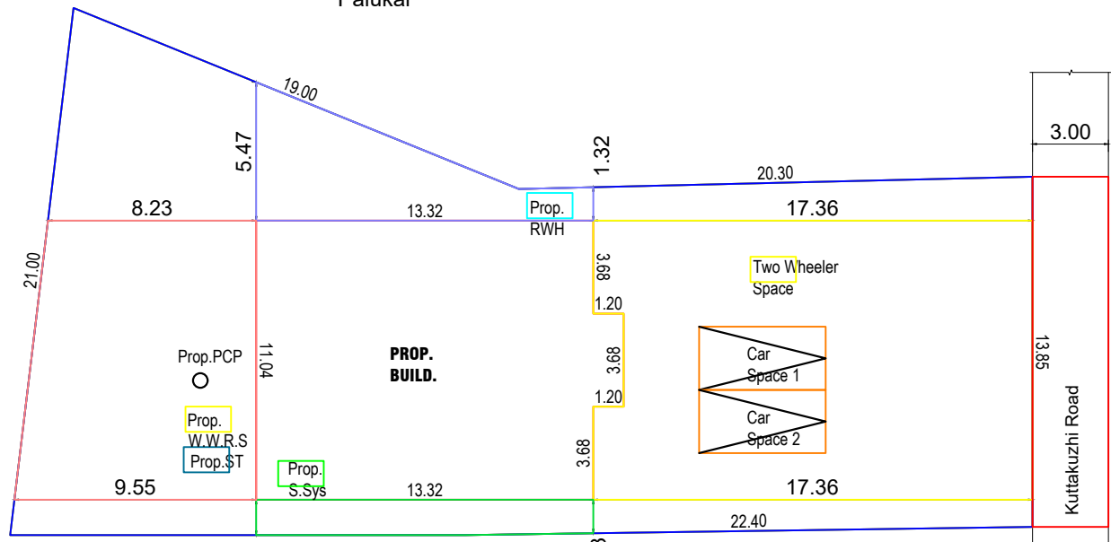
SITE PLAN SCALE : 1:100
