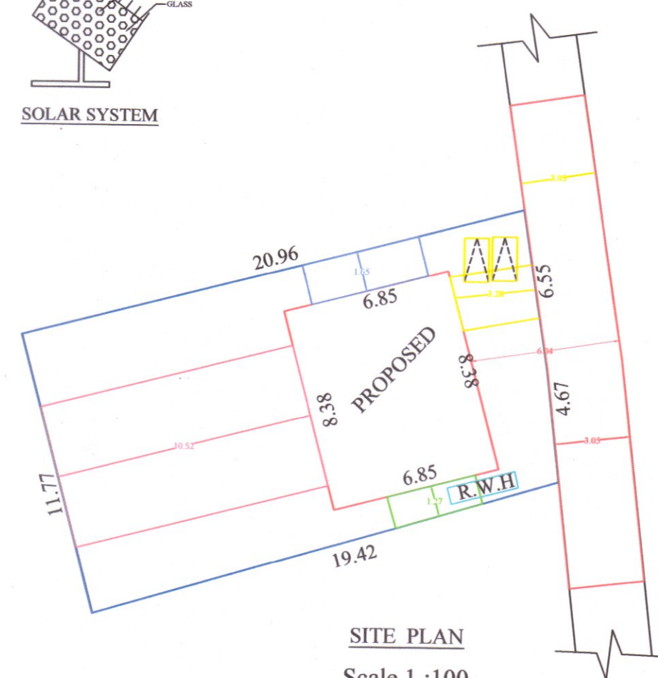
Scale 1 : 100
