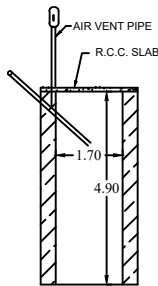
SOAK PIT
