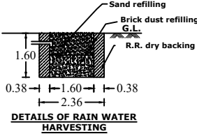
SOAK PIT
