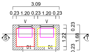
TOILET PLAN
