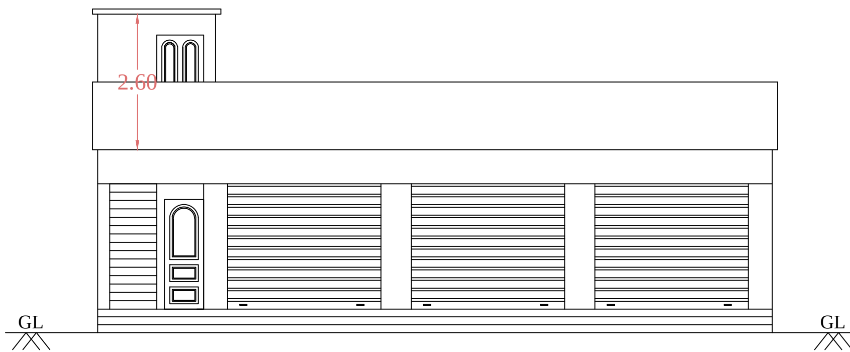
ELEVATION
