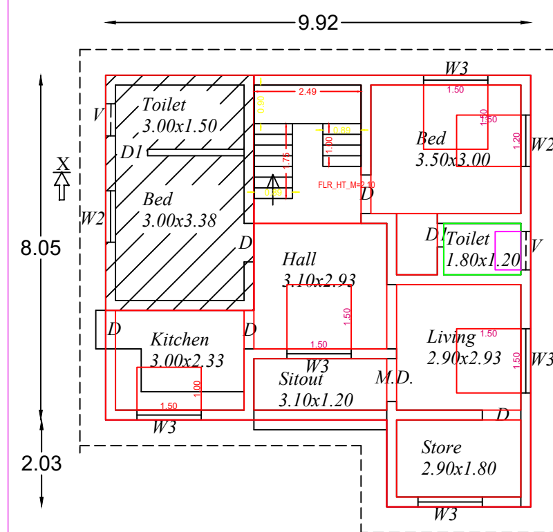
6 ————— 3.36 ————— 2 FLOOR PLAN
