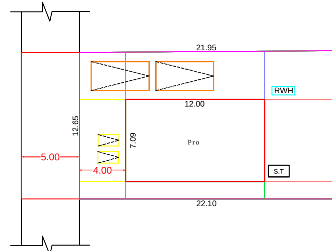
SCALE 1:100 SITE PLAN
