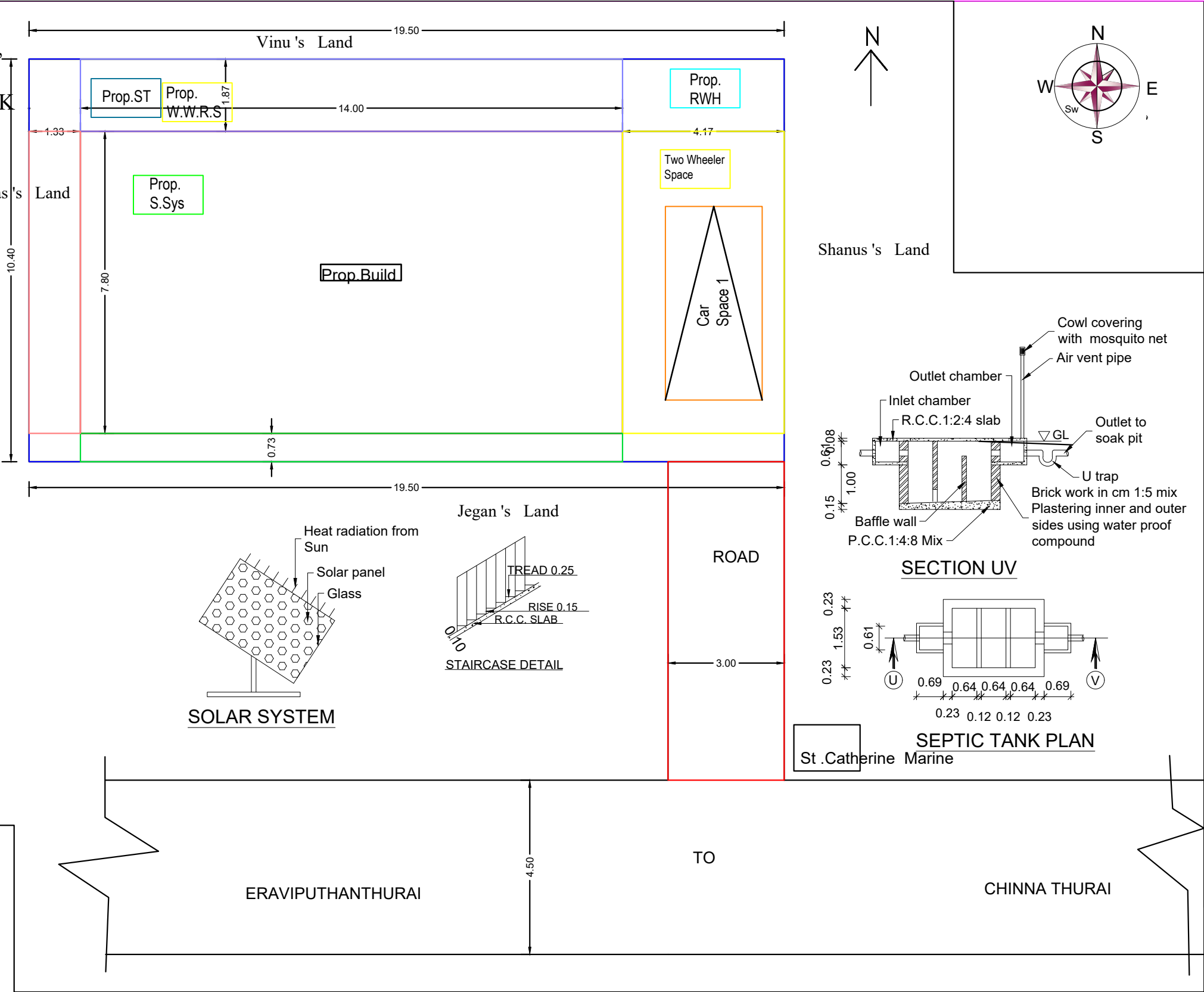
KEY PLAN SCALE 1 : 100
