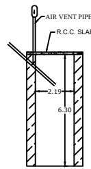
SOAK PIT
