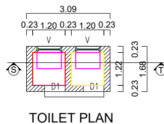
TOILET PLAN
