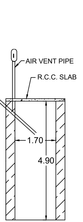
SOAK PIT
