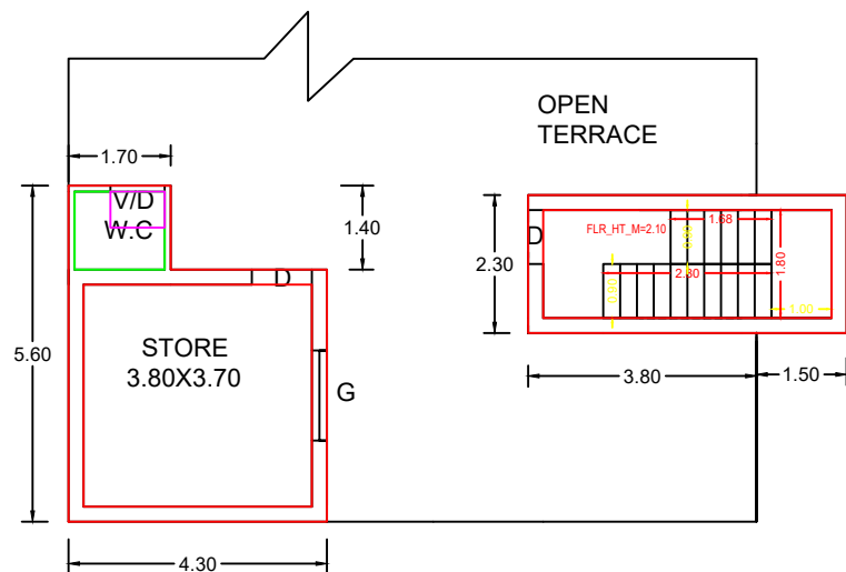
S.F. PLAN
