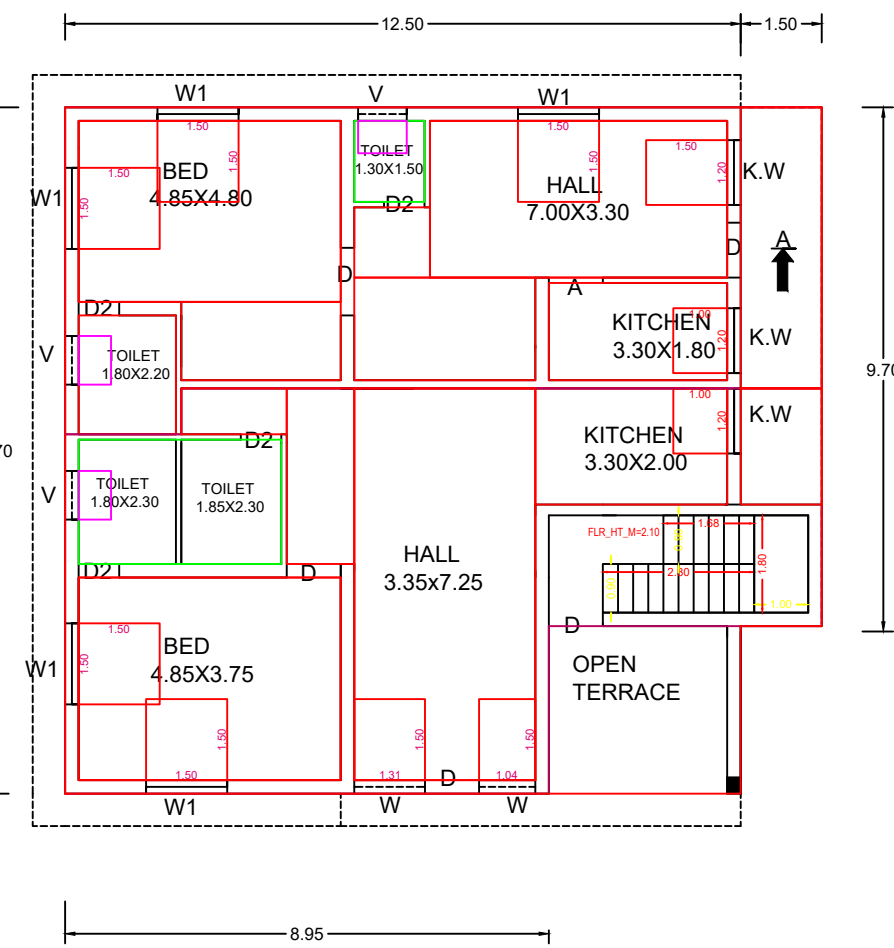
F.F. PLAN
