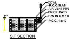
S.T SECTION
