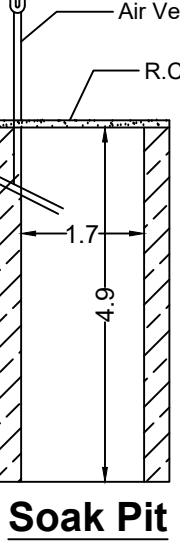
Soak Pit
