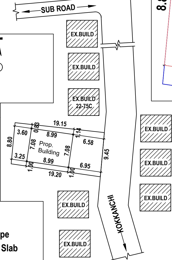
KEY PLAN SCALE : 1:400
