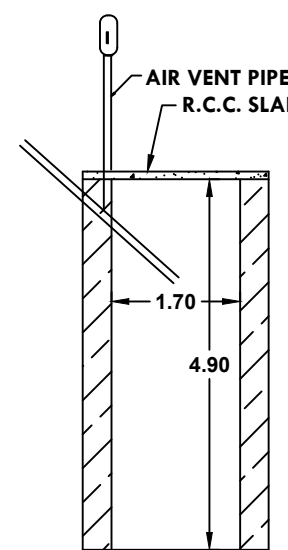
SOAK PIT
