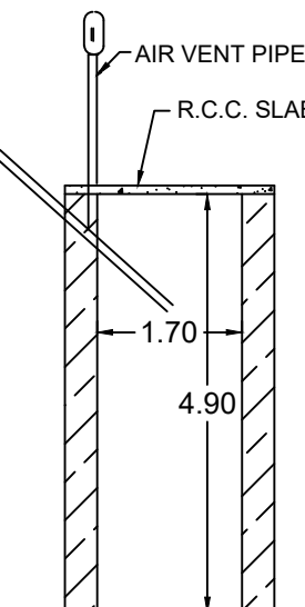
SOAK PIT
