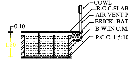
S.T SECTION
