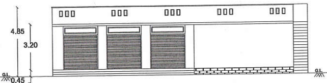
ELEVATION
