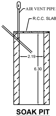
SOAK PIT
