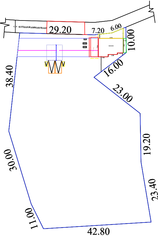
SITE PLAN SCALE 1:400
