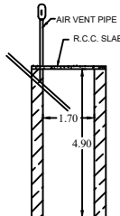
SOAK PIT
