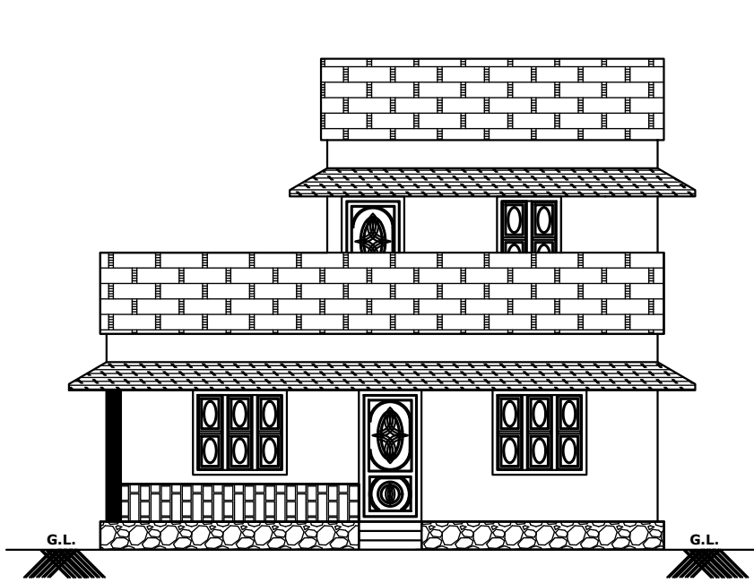
ELEVATION
