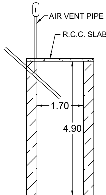
SOAK PIT
