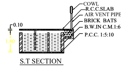
S.T SECTION
