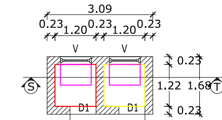
TOILET PLAN
