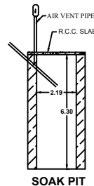
SOAK PIT
