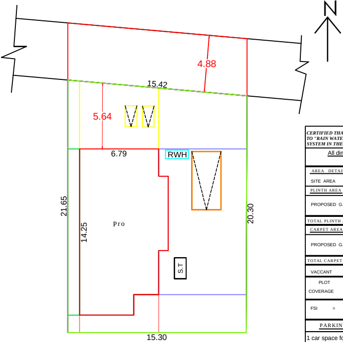
SCALE 1:100 SITE PLAN
