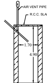
SOAK PIT
