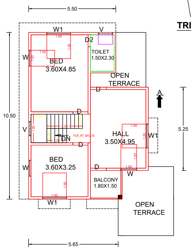
F.F. PLAN
