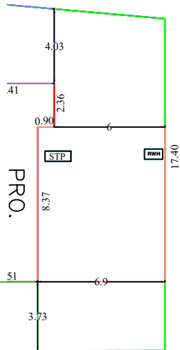
SITE PLAN SCALE 1:100
