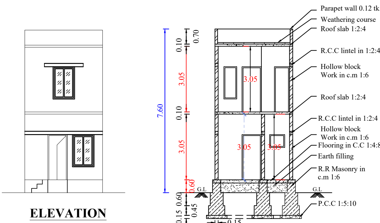
ELEVATION
