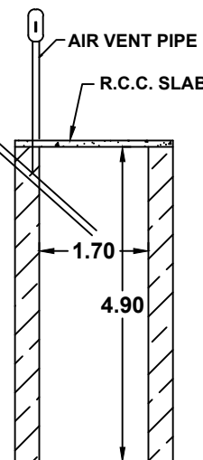
SOAK PIT
