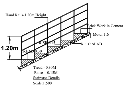
Scale:1:500
