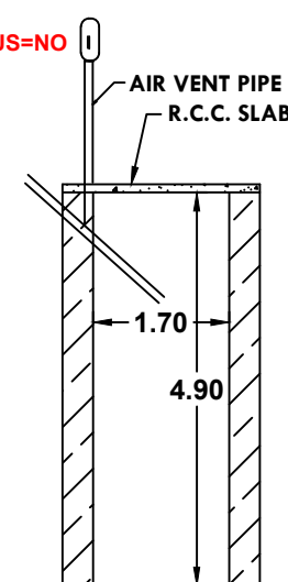
SOAK PIT
