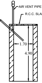
SOAK PIT
