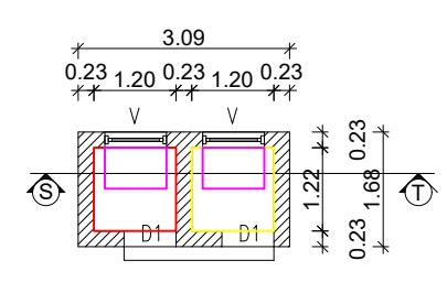
TOILET PLAN
