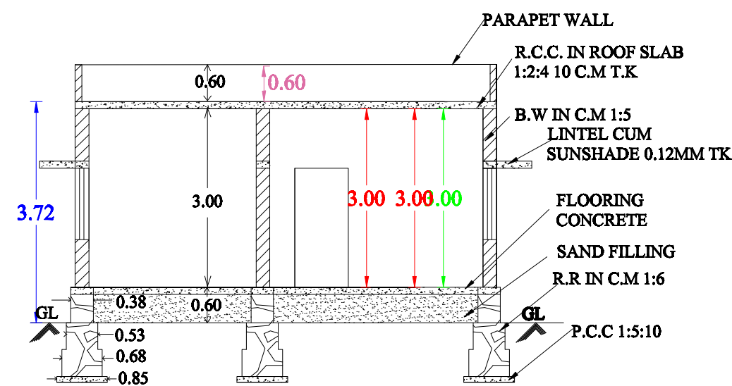
SECTION A-B
