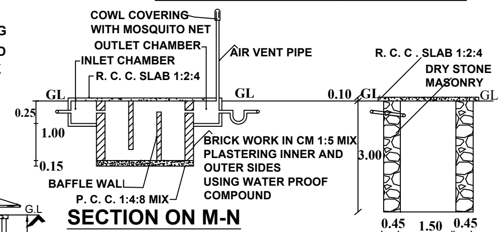
SOAK PIT
